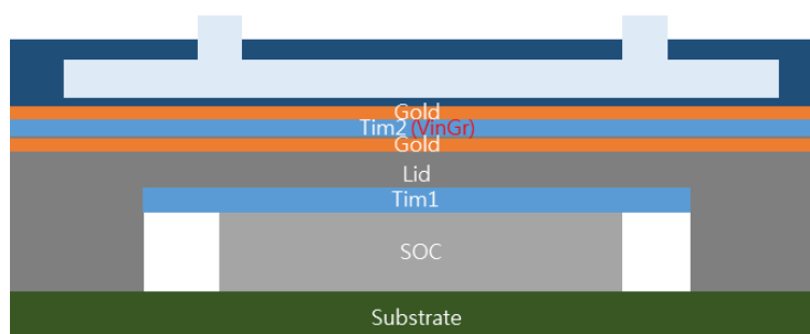
圖 3：鍍金水冷板示意圖
